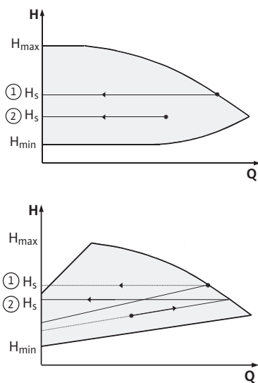
Рис. 40: Регулирование Δp-с/Δp-в
