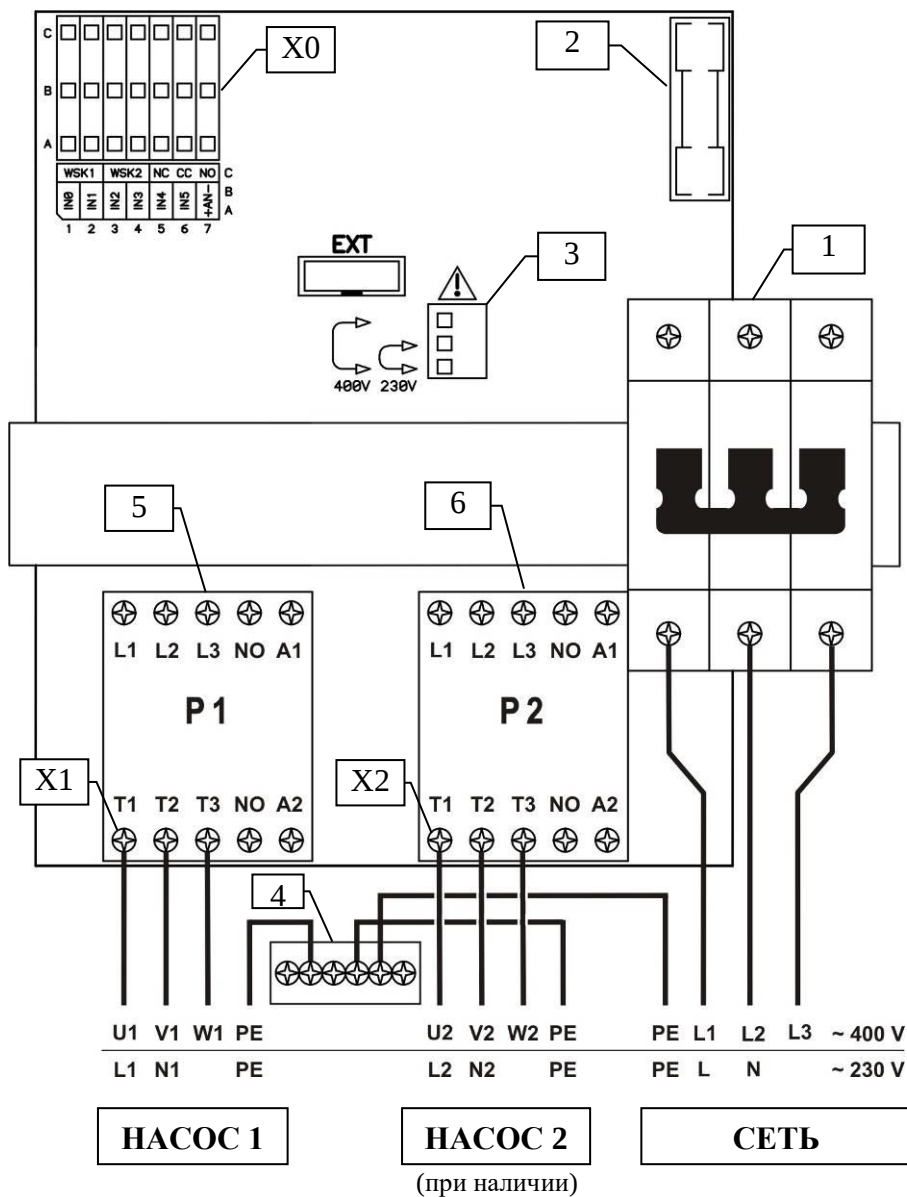
Рис. 1 Внутренний вид прибора и подсоединение сетевых контактов
